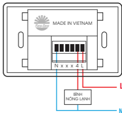
Sơ đồ nối dây cho công tắc bình nóng lạnh
