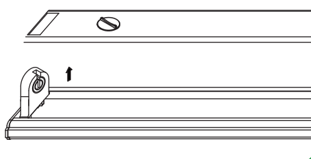
Bước 5: Lắp nắp máng đèn - Lắp tube led
