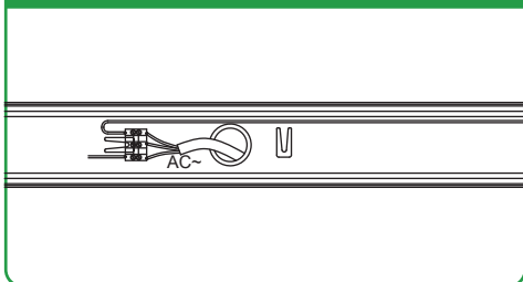
Bước 4: Đấu nối máng đèn với nguồn điện
