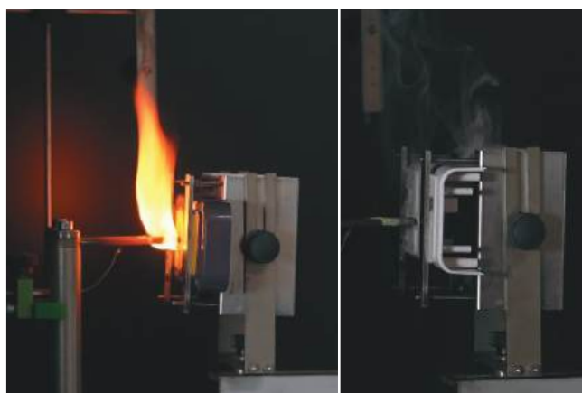
Kiểm tra khả năng chịu cháy bộ vỏ
